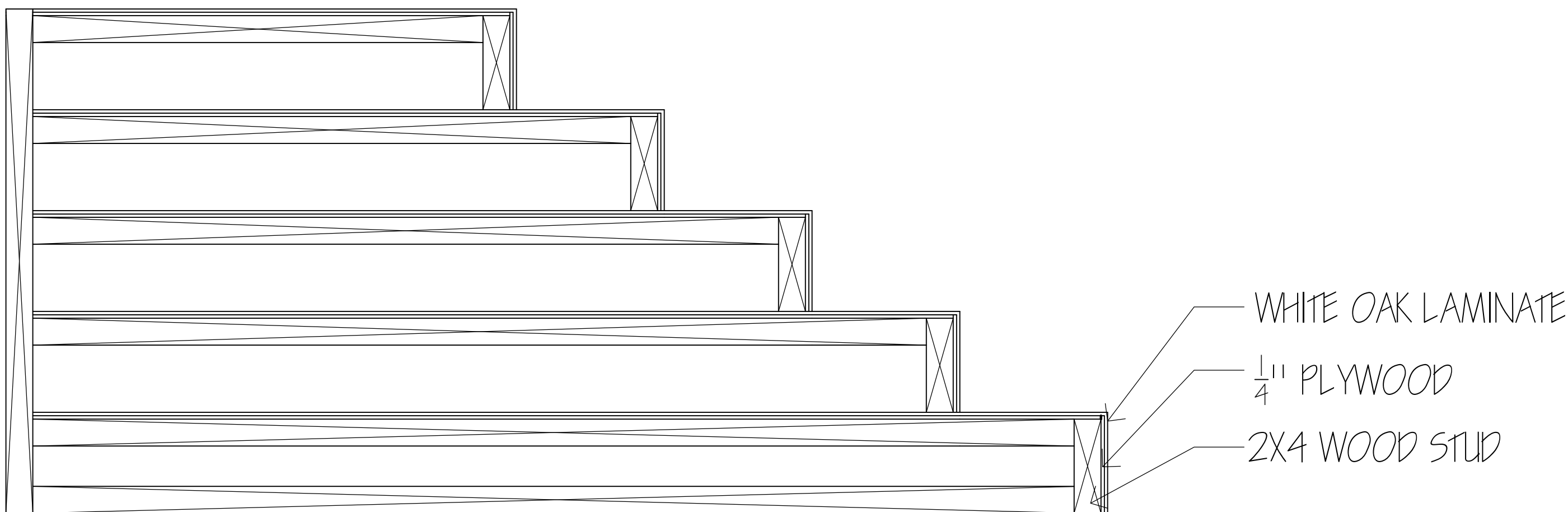
2 LOBBY STAIR SECTION SCALE: 1/2" = 1'-0"
