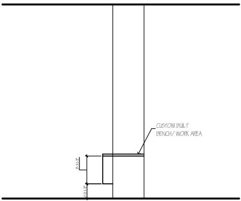
7 COLUMN ELEVATION SCALE: 1/4" = 1'-0"
