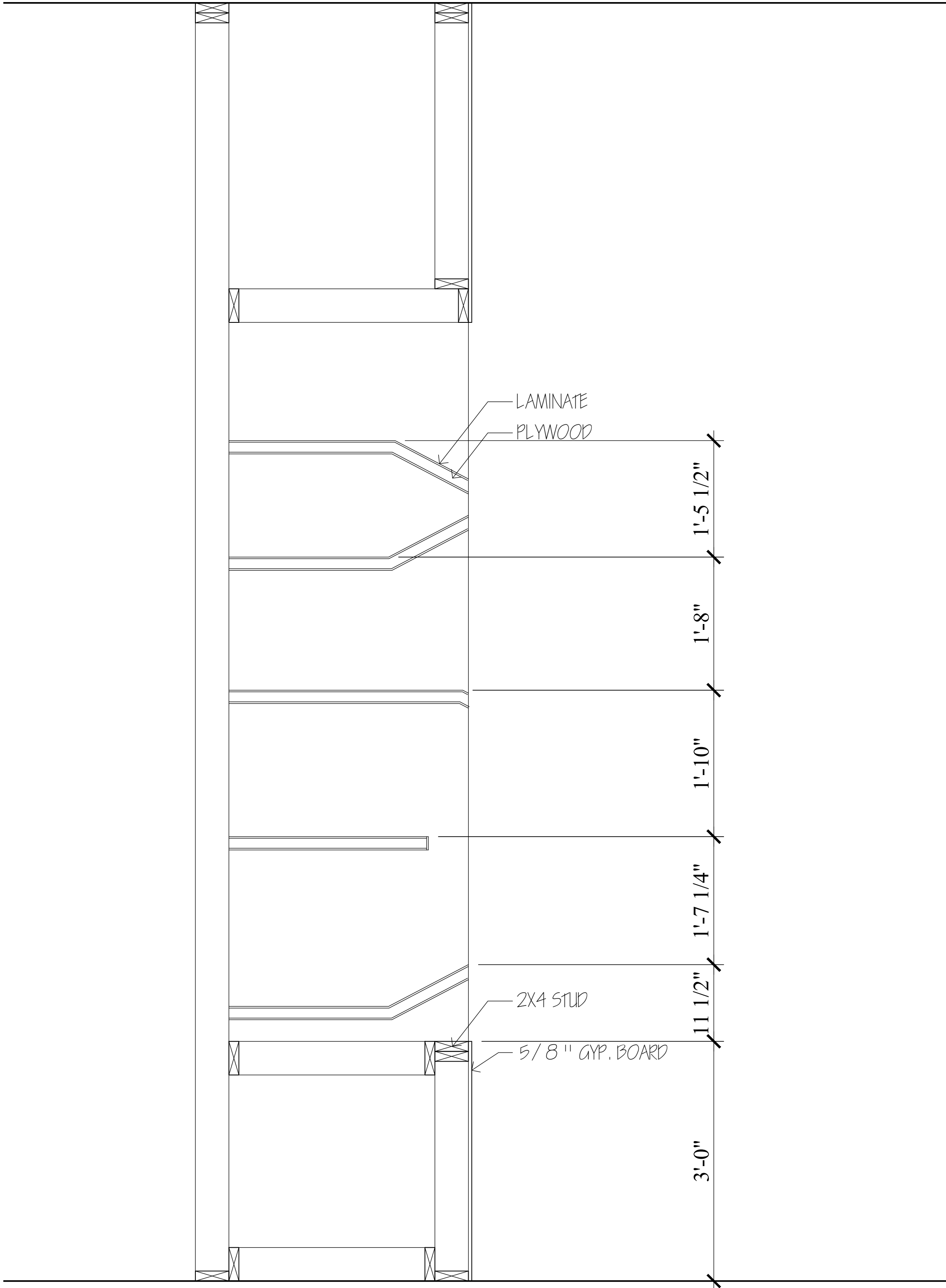
6 SHOWCASE SECTION SCALE: 1" = 1'-0"
