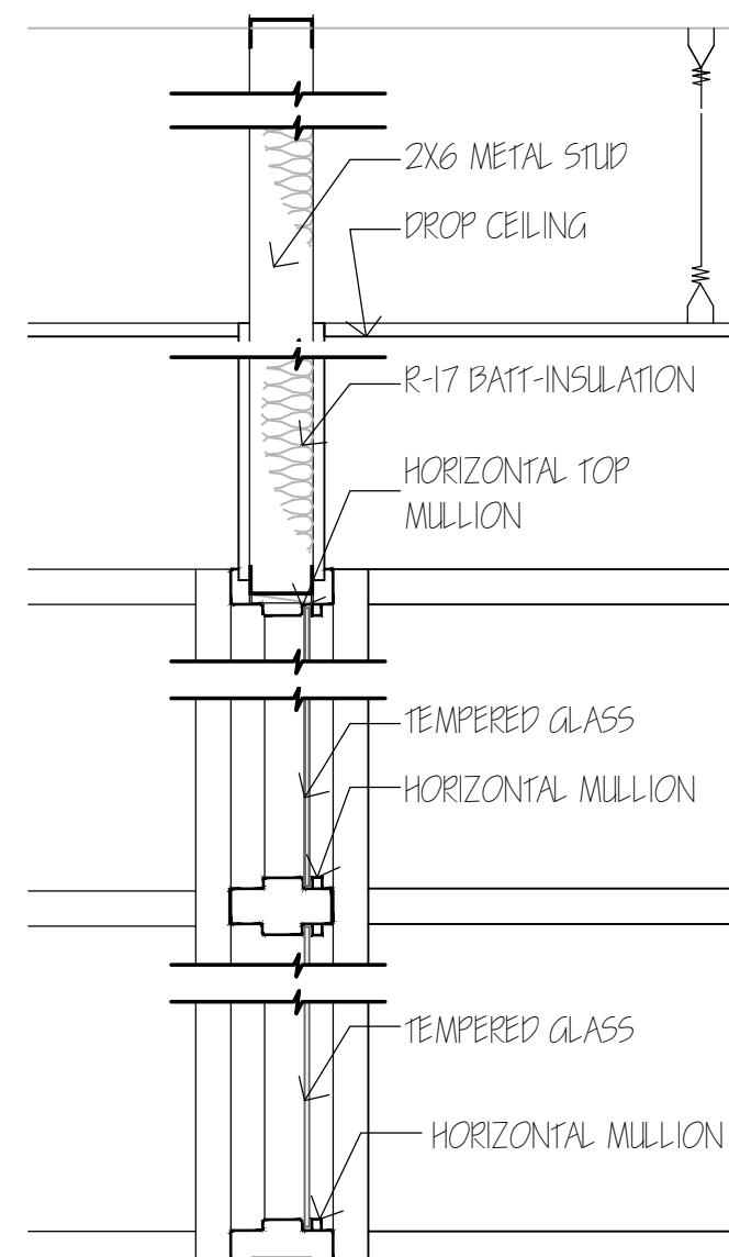
2 PARTITION TYPE SCALE: N.T.S.
