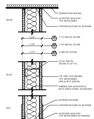
1 PARTITION TYPE SCALE: N.T.S.
